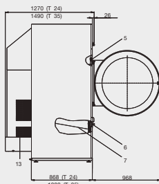
ZEZADU T 24 35 (PLYNOVÝ MODEL)
