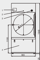
ZEZADU T 24 35 (PARNÍ MODEL)
